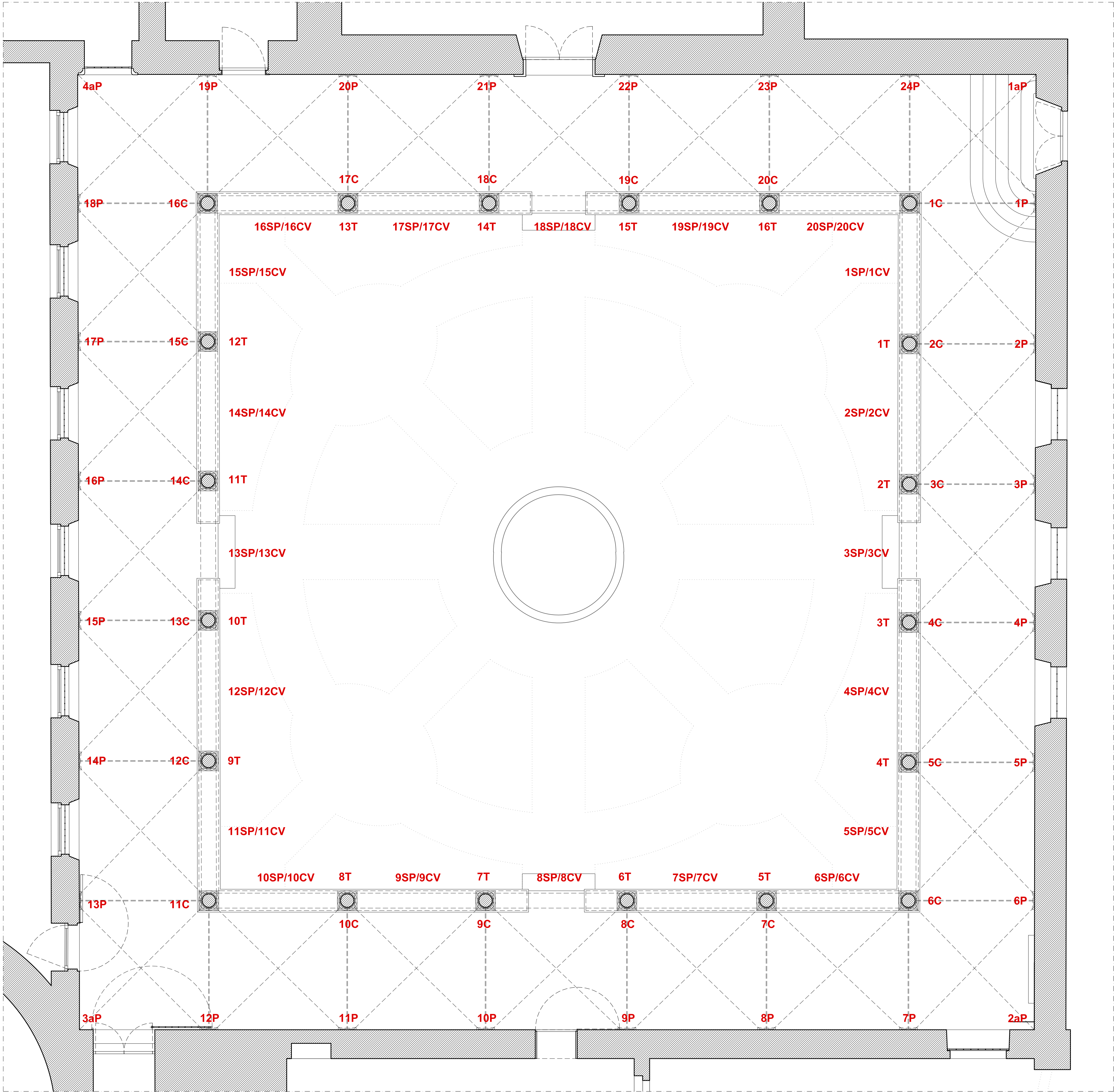
Pianta (sezione +80cm.) scala 1:50
